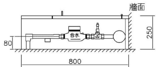
側面圖
