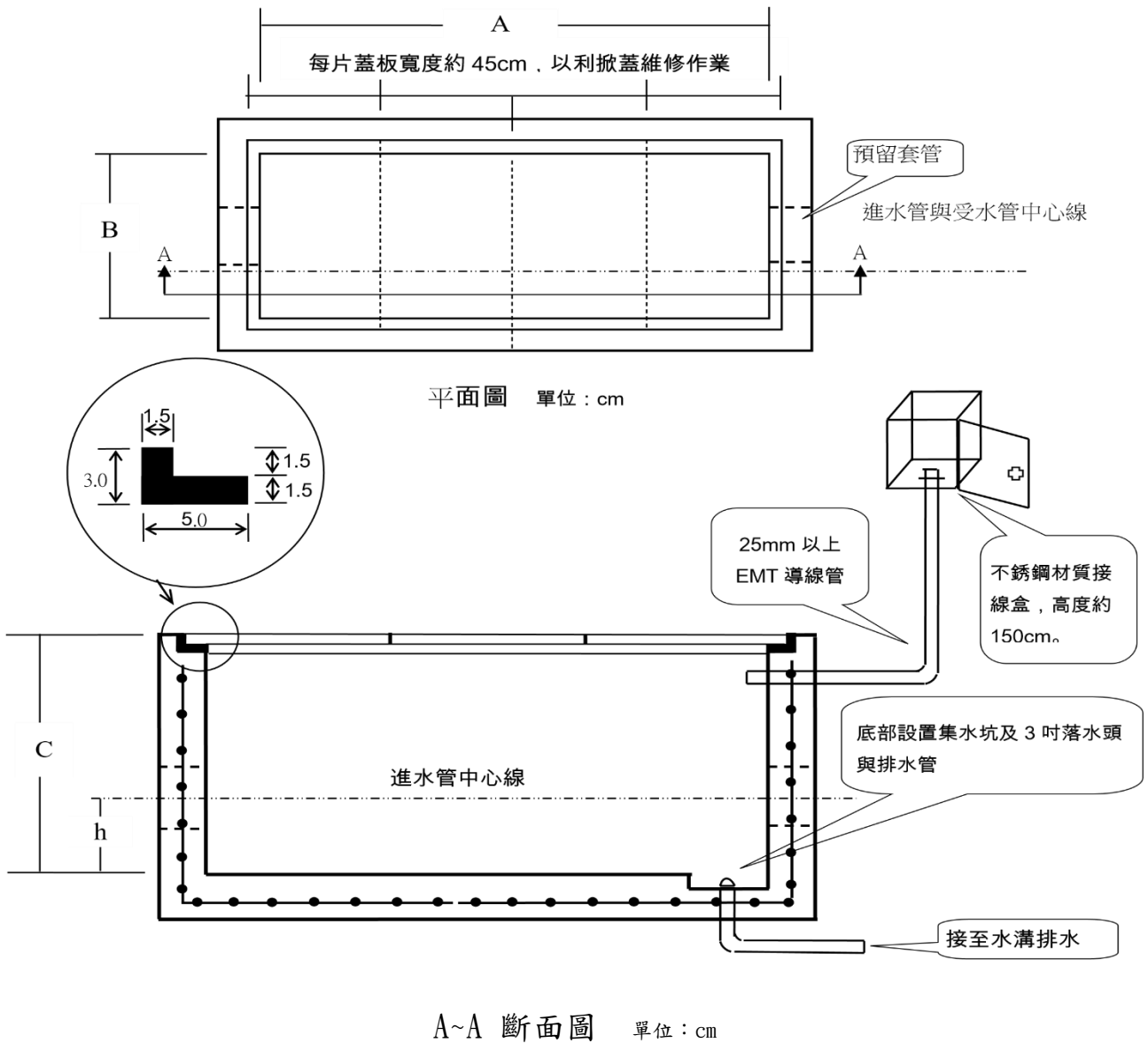
口徑 50mm ~ 150mm 水量計箱(窰井)參考尺寸
