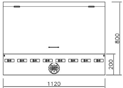
上視圖
